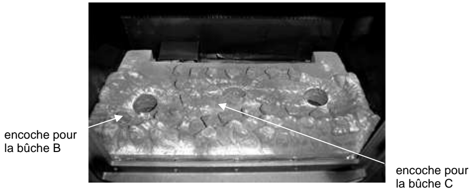
Brûleur céramique
